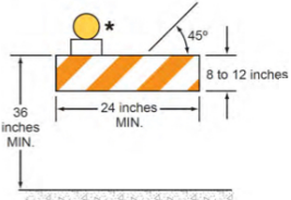
TYPE 1 BARRICADE **
